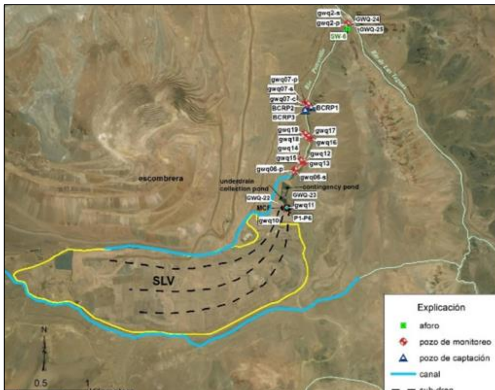
Ilustración 1-11. Sistema de bombeo y monitoreo BCRP
