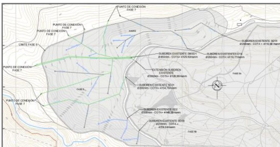
Ilustración 1-45. Sistema de subdrenaje
