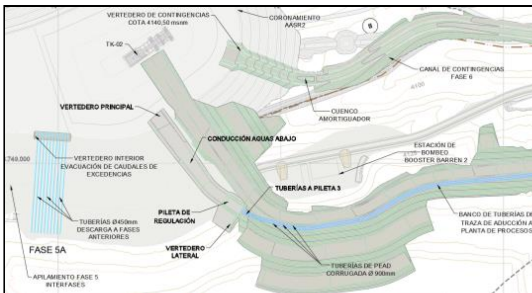
Ilustración 1-43. Esquema sistema de evacuación de caudales de excedencias
