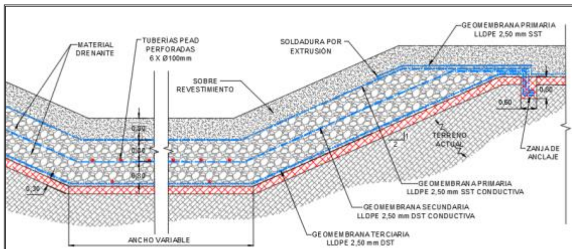
Ilustración 1-50. Detalle del SRRF2 dentro del AASR2.
