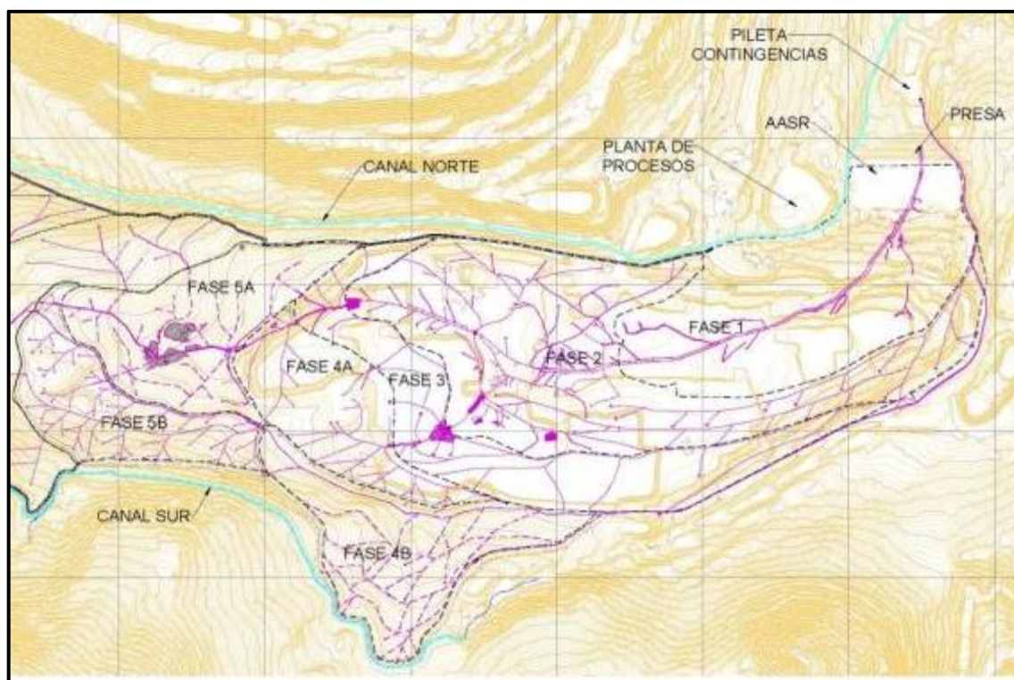
Ilustración 1-8 Sistema de subdrenaje -Fases 1 a 5
