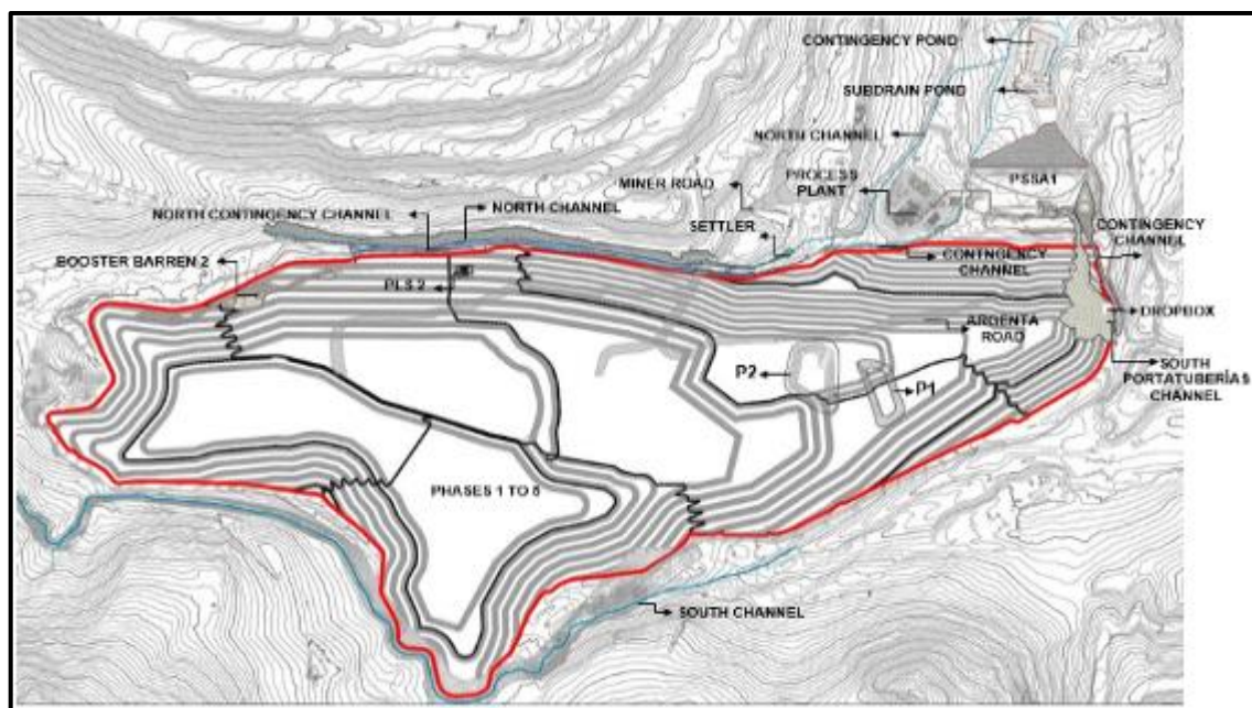
Ilustración 1-34. Apilamientos fases 1 a 5 SLV
