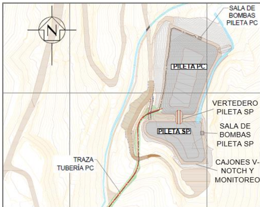
Ilustración 1-15. Vinculación entre piletas SP y PC
