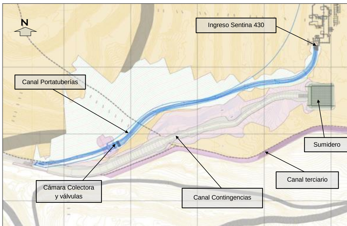
Ilustración 1-29. Obras Canal Portatuberías Sur
