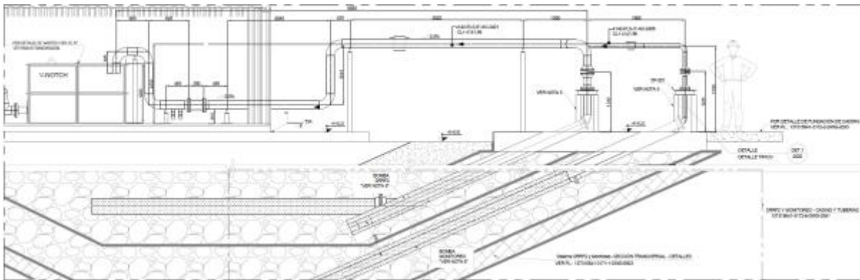
Ilustración 1-48. Sistema de bombeo SRRF2
