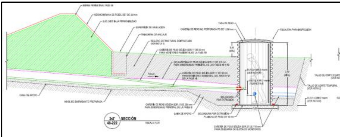
Ilustración 1-10 Detalle Buzón de monitoreo
