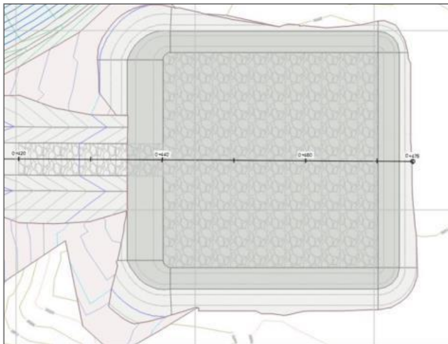
Ilustración 1-30. Planta sumidero
