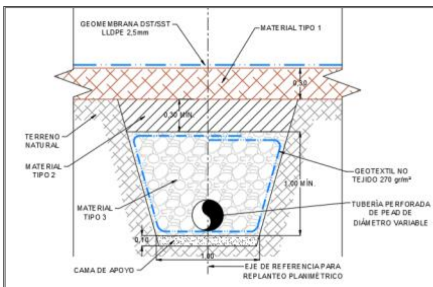
Ilustración 1-46. Detalle tipo de zanja del sistema de subdrenaje
