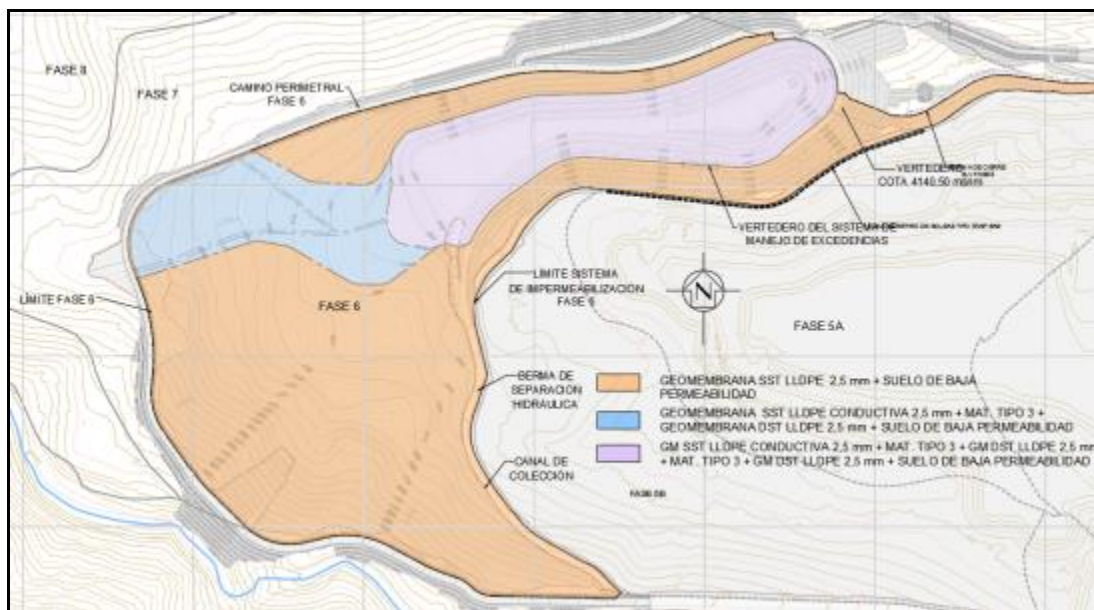
Ilustración 1-52. Sistema de revestimiento fase 6
