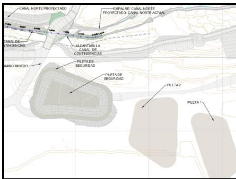
Ilustración 1-44. Ubicación de pileta 3 de emergencia y piletas 1 y 2
