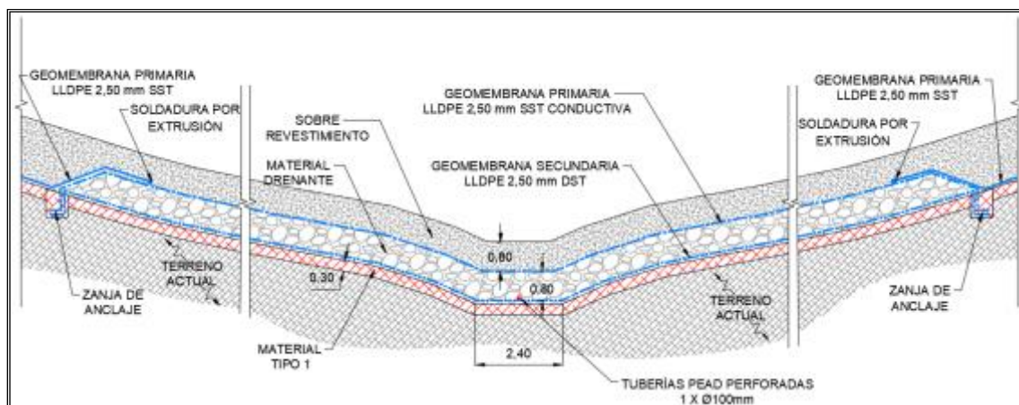
Ilustración 1-51. Detalle del SRRF2 fuera del AASR2.
