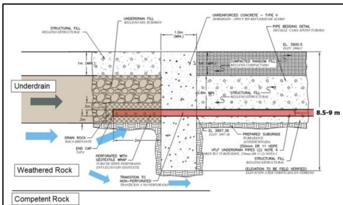
Ilustración 1-17. Muro corta fugas
