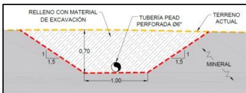
Ilustración 1-38. Detalle de zanja de infiltración Norte
