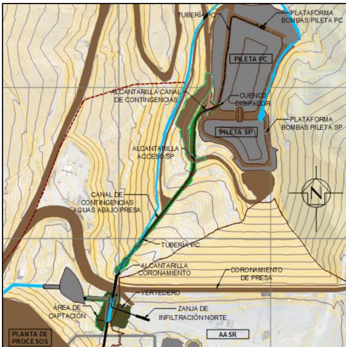
Ilustración 1-37. Sistema bombeo desde pileta PC
