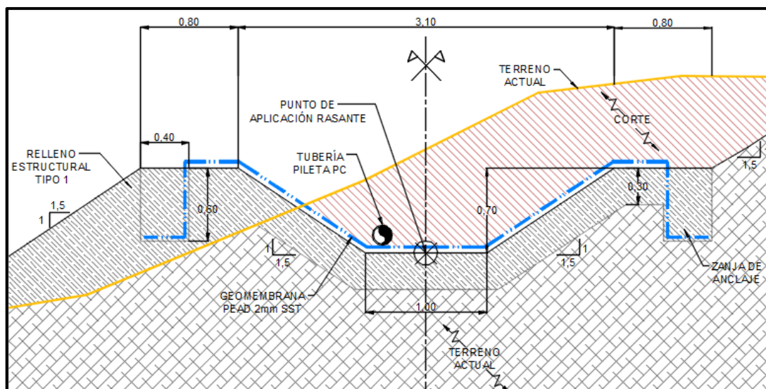
Ilustración 1-36. Sección tipo del canal de contingencias aguas abajo vertedero AARS1
