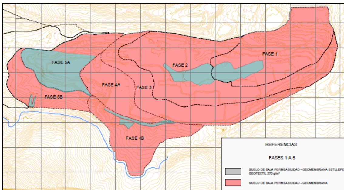
Ilustración 1-20. Sistema de revestimiento - Fase 1 a 5
