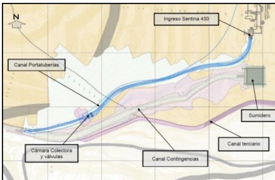
Ilustración 1-22. Configuración general canal portatuberías Sur
